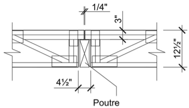
DÉTAIL # 1
