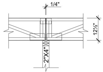
DÉTAIL # 3
