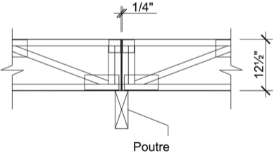
DÉTAIL # 1
