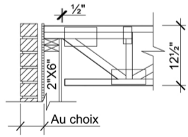
DÉTAIL # 2
