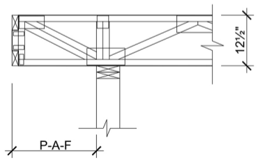
DÉTAIL # 6
