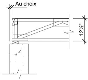
DÉTAIL # 2
